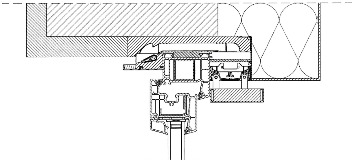
Rys. F4. Przykładowy schemat montażu nawiewnika INSOLIO z czerpnią w wariacie NDF (z filtrem i tłumikiem akustycznym)
