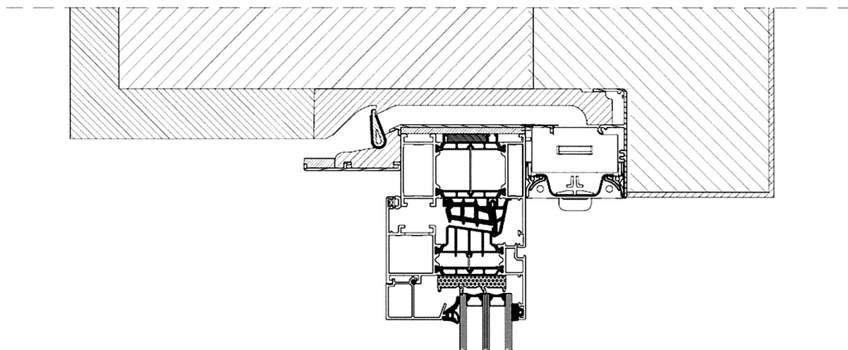
Rys. F1. Przykładowy schemat montażu nawiewnika INSOLIO z pompą w wariantcie E (z siatką)
