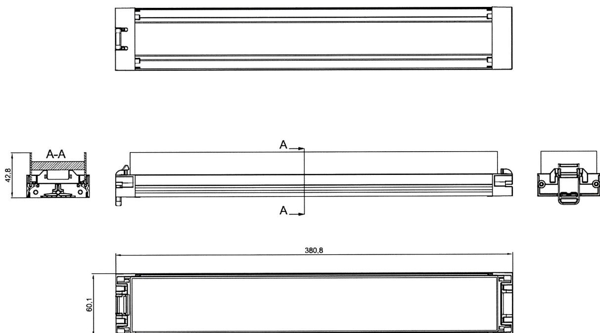
Rys. A4. Czerpnia powietrza zewnętrznego nawiewnika INSOLIO, wariant F z filtrem (wymiary w mm)
