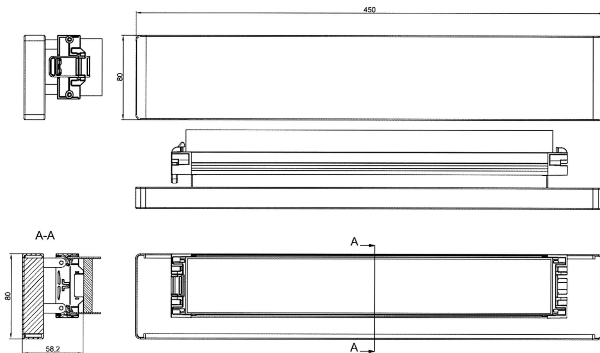
Rys. A6. Czerpnia powietrza zewnętrznego nawiewnika INSOLIO, wariant NDF z filtrem i tłumikiem akustycznym (wymiary w mm)
