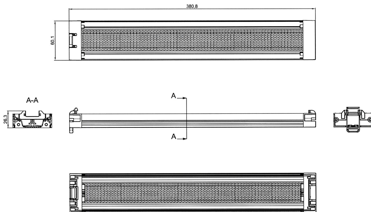
Rys. A3. Czerpnia powietrza zewnętrznego nawiewnika INSOLIO, wariant E z siatką (wymiary w mm)
