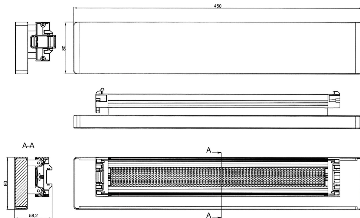
Rys. A5. Czerpnia powietrza zewnętrznego nawiewnika INSOLIO, wariant ND z siatką i tłumikiem akustycznym (wymiary w mm)
