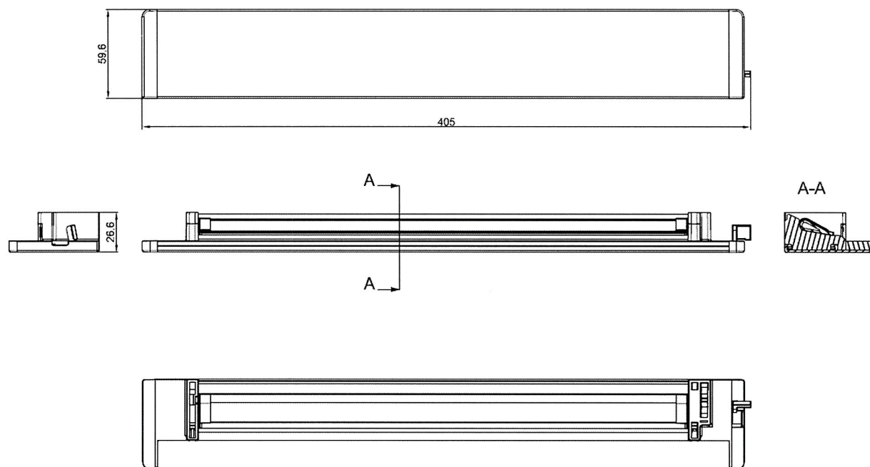
Rys. A1. Regulator przepływu powietrza nawiewnika INSOLIO (wymiary w mm)
