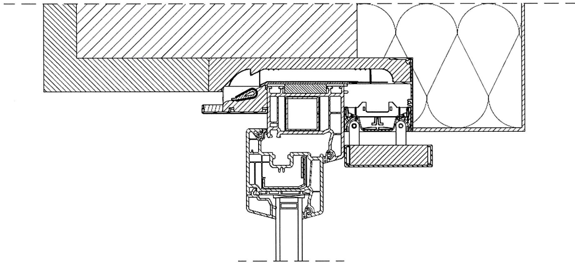
Rys. F3. Przykładowy schemat montażu nawiewnika INSOLIO z czerpnią w wariacie ND (z siatką i tłumikiem akustycznym)
