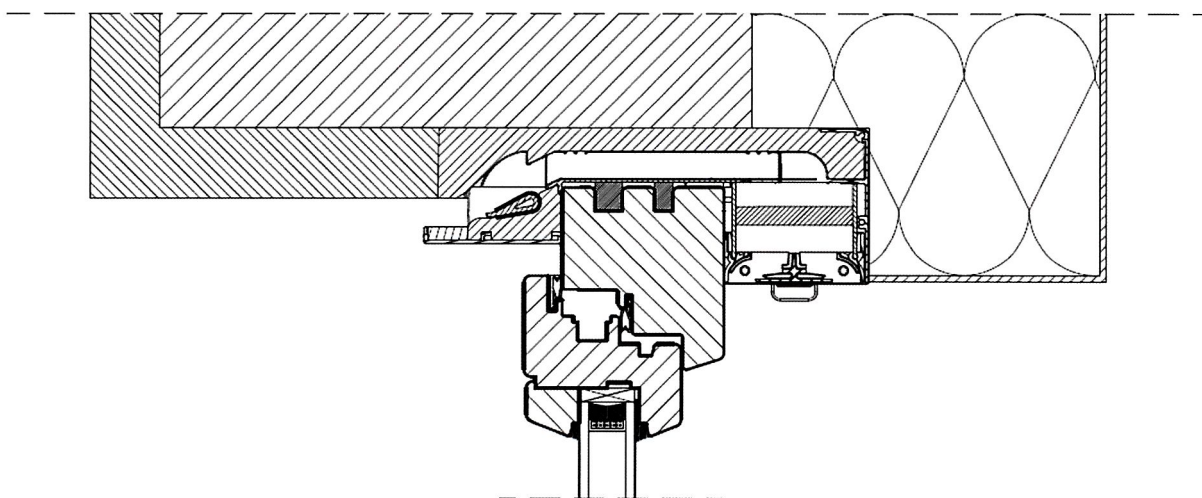
Rys. F2. Przykładowy schemat montażu nawiewnika INSOLIO z pompą w wariantcie F (z filtrem)
