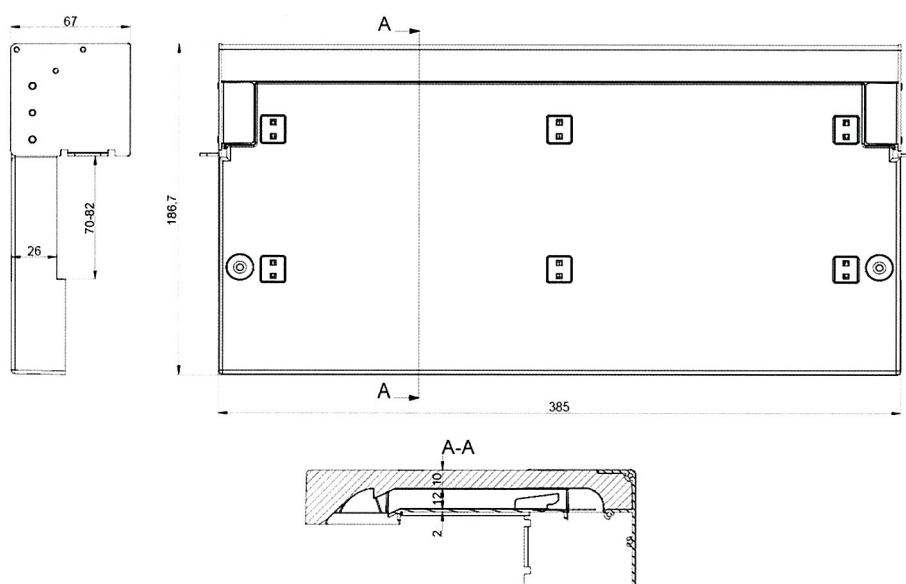
Rys. A2. Kanał przelotowy nawiewnika INSOLIO (wymiary w mm)
